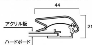
フレーム幅44mmの角Rタイプ
