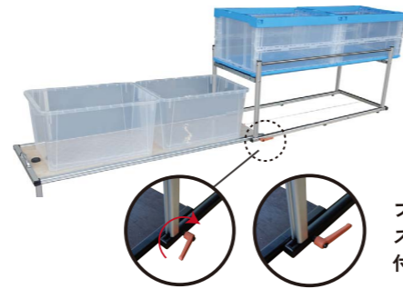
面板を引き出す際は スライドパイプを取り付けて下さい
